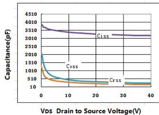
图 6.典型电容与漏源电压的曲线
