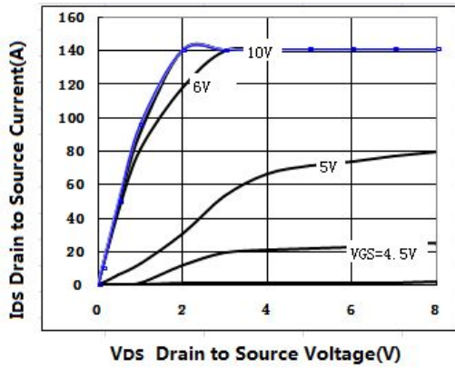
图 1 输出特性曲线, T_c=25^\circ C
