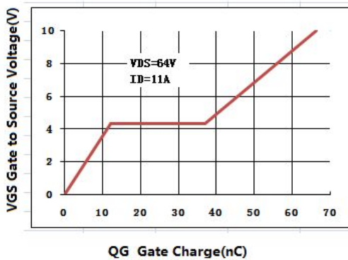
图 5 典型栅极电荷与栅源电压曲线
