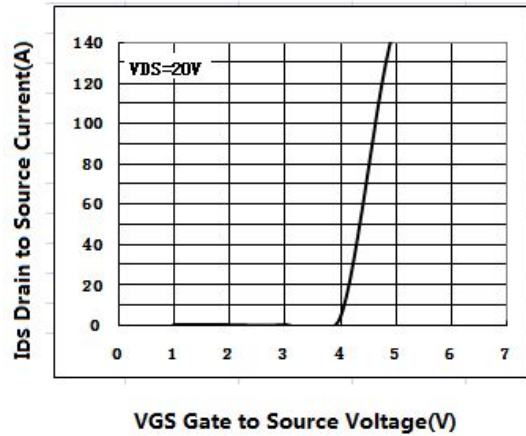
图 4 转移特性曲线
