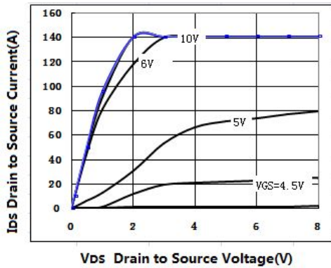
图 1 输出特性曲线, T_c=25^\circ C
