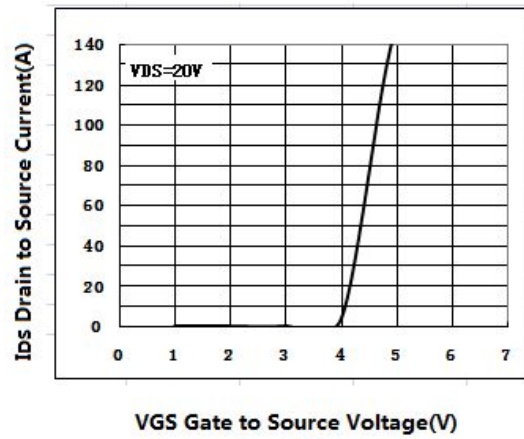
图 4 转移特性曲线
