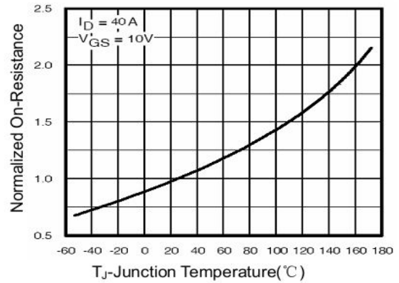
图 4 导通电阻与结温度曲线
