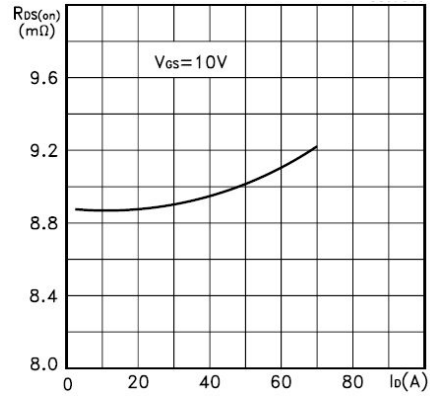
图 2 导通电阻与漏极电流的曲线
