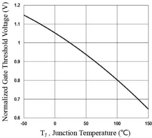
图 3 归一化开启电压与结温关系曲线 Fig.3 Normalized Vth vs. Tj
