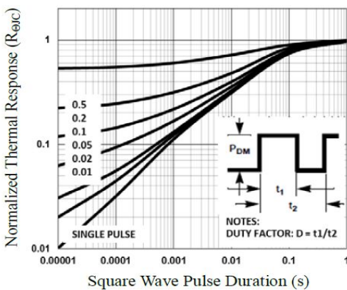
图 5 归一化阻抗 Fig.5 Normalized Transient Impedance
