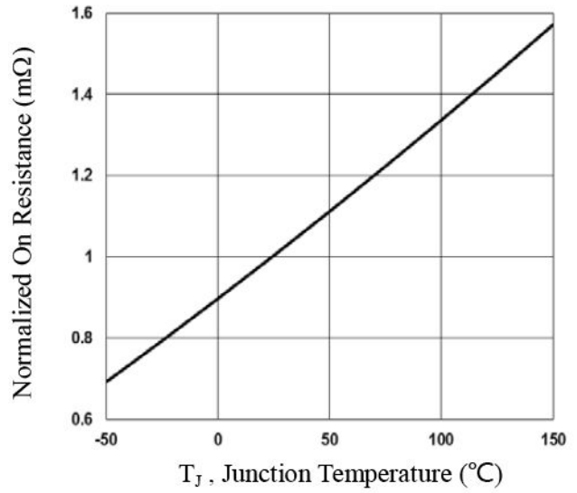
图 2 归一化导通电阻与结温关系曲线 Fig.2 Normalized RDSON vs. Tj
