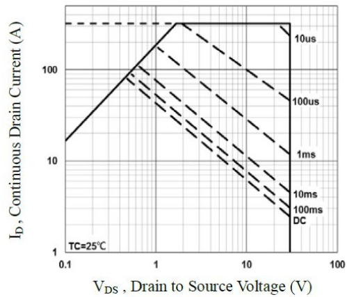
图 6.最大安全工作区 Fig.6 Maximum Safe Operation Area
