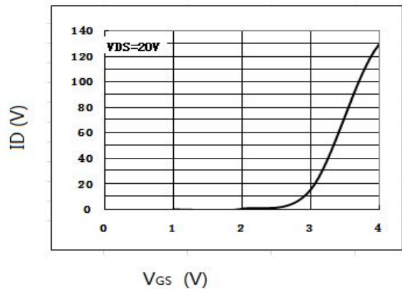
图 4 转移特性曲线
