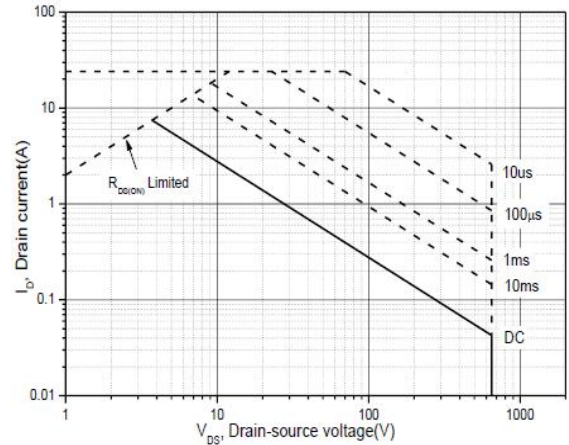
图 2 最大安全工作区曲线 (TO-220FP) Fig2 Maximum Safe Operating Area
