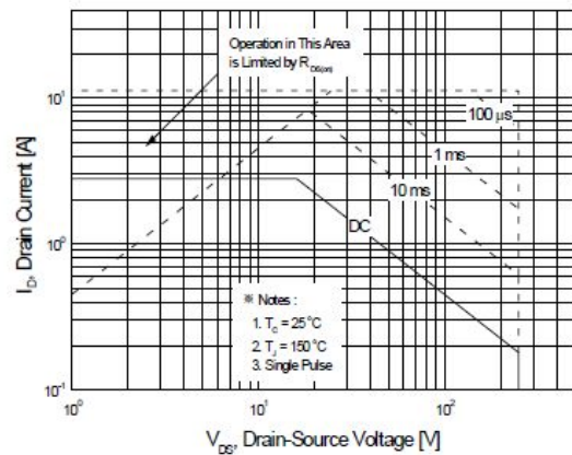
图 6 最大安全工作区曲线
