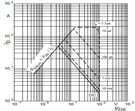
图 6 最大安全工作区曲线&TO-220
