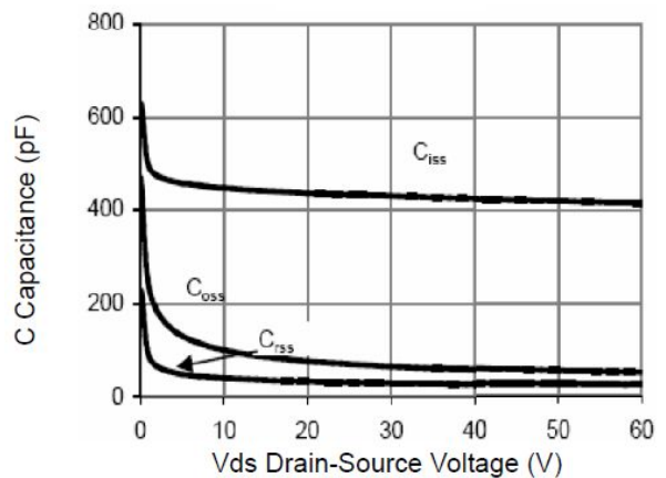
Figure 6: Capacitance vs V_{DS} 图 6. 电容与漏源电压的曲线
