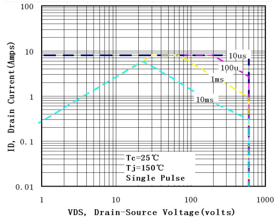
图 6-2 SIF2N60F (TO-220FP)
