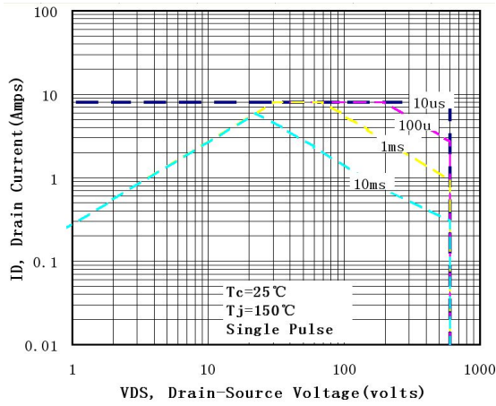
图 6-1 SIF2N60F (TO-220)
