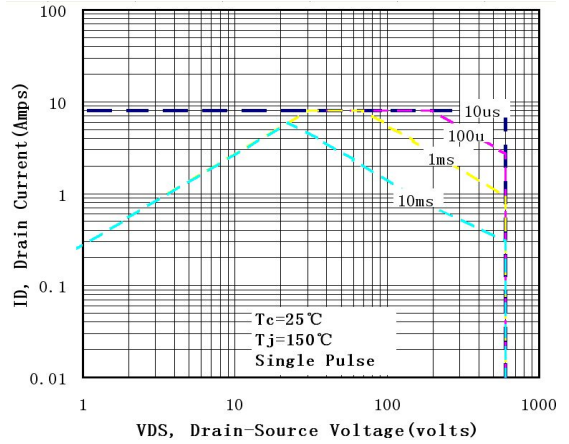
图 6-2 SIF2N60D (TO-220FP(L))
