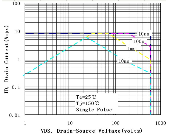
图 6-2 SIF2N60C(TO-220FP)
