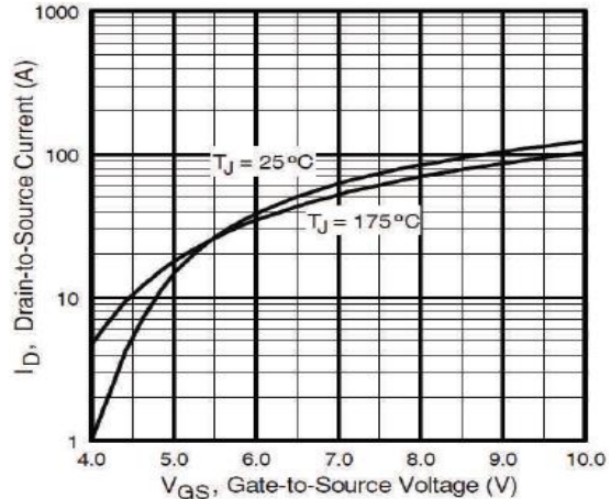
图 2 典型转移特性曲线
