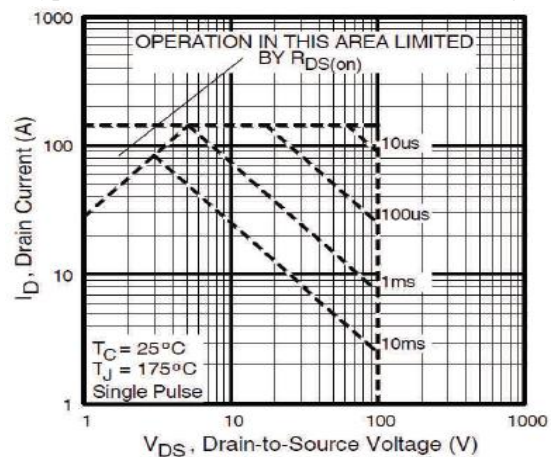
图 6 最大安全工作区曲线&TO-251&252
