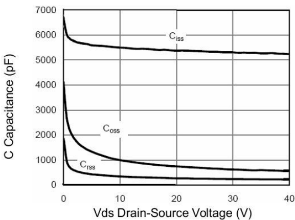
图 5 电容曲线
