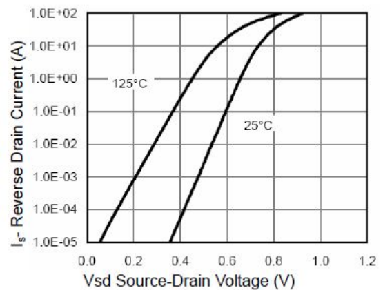
图 6.二极管正向曲线
