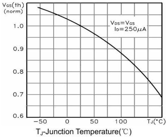
图 3 归一化开启电压与结温关系曲线
