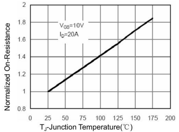
图 2 归一化导通电阻与结温关系曲线
