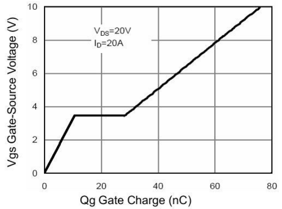
图 4 栅电荷波形
