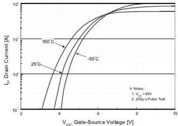
图 2 转移特性
