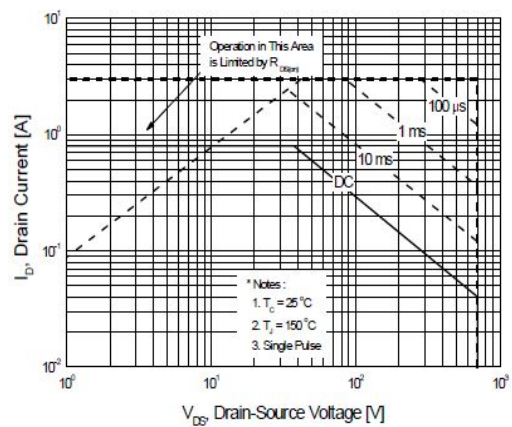
图 6 最大安全工作区曲线
