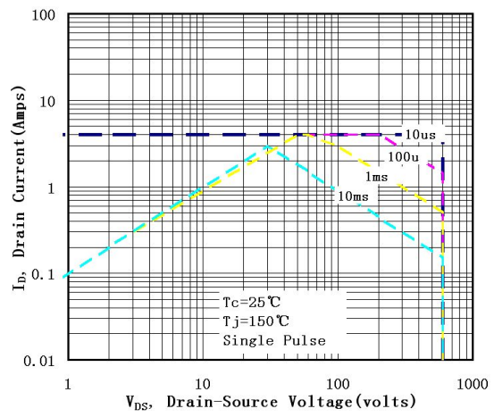
图 6-2 SIF1N65F(TO-251T&251S&252(T))
