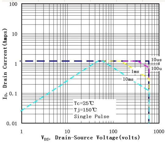
图 6-1 SIF1N65F(TO-92)
