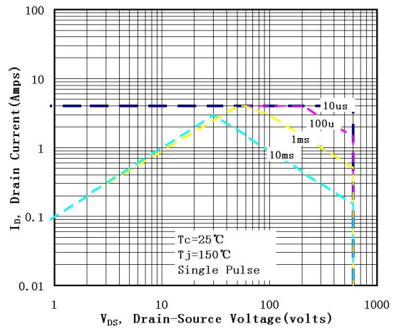
图 6-2 SIF1N60(TO-251T&251S&252(T))
