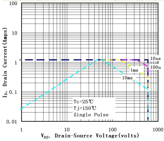
图 6-1 SIF1N60(TO-92)
