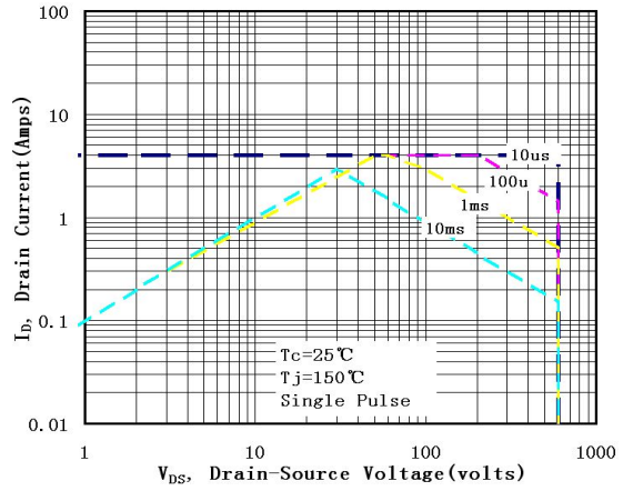
图 6-2 SIF1N60F(TO-251&251S&252(T))
