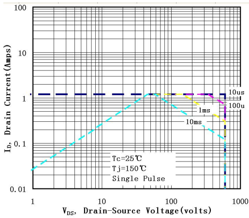
图 6-1 SIF1N60F(TO-92)
