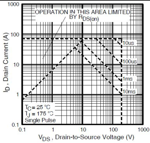
图 7 最大安全工作区曲线&TO-220 Fig7 Maximum Safe Operating Area&TO-220
