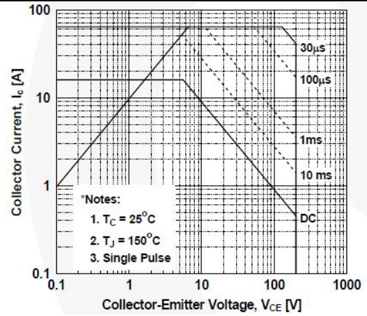
图 8 最大安全工作区曲线&TO-220FP Fig8 Maximum Safe Operating Area&TO-220FP
