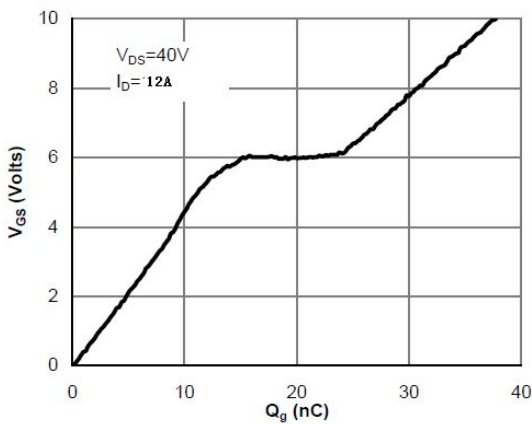
图 5 典型栅极电荷与栅源电压曲线
