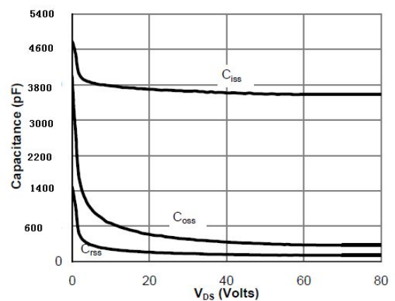
图 6. 典型电容与漏源电压的曲线
