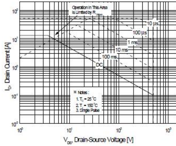
图 6-2 SIF11N50F(TO-220FP(L)) 最大安全工作区曲线 Fig6-2 Maximum Safe Operating Area
