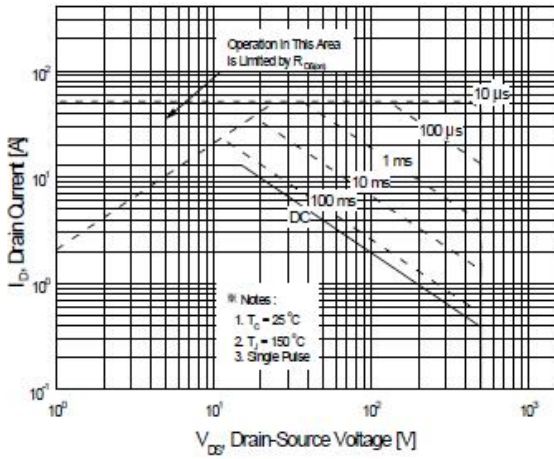
图 6-1 SIF11N50F(TO-220) 最大安全工作区曲线 Fig6-1 Maximum Safe Operating Area
