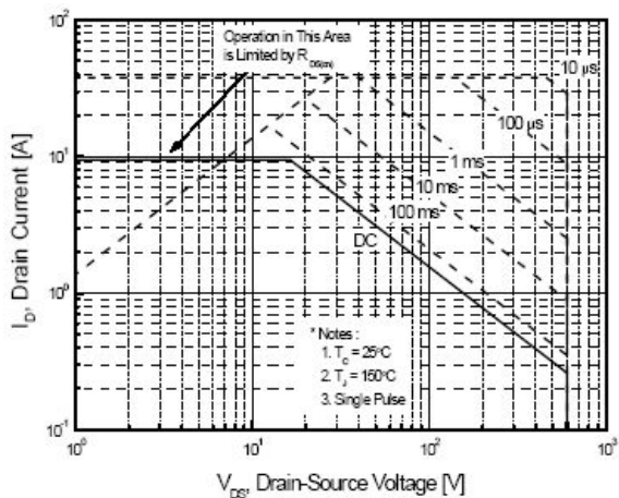
图 6-1 SIF10N65EA(TO-220)
