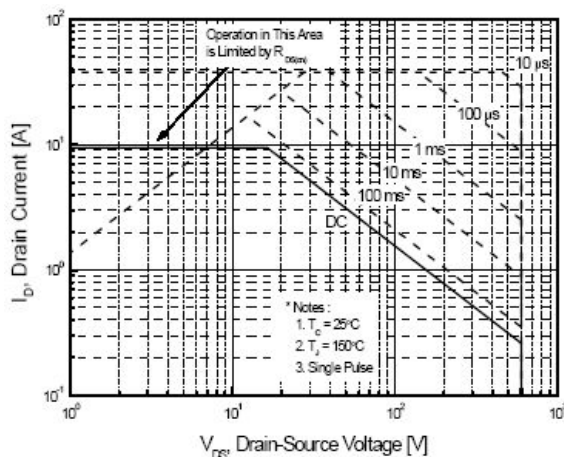
图 6-1 SIF10N65EA(TO-220FP)
