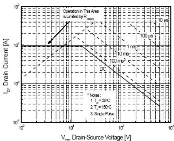
图 6-3 SIF10N60C(TO-262&263)
