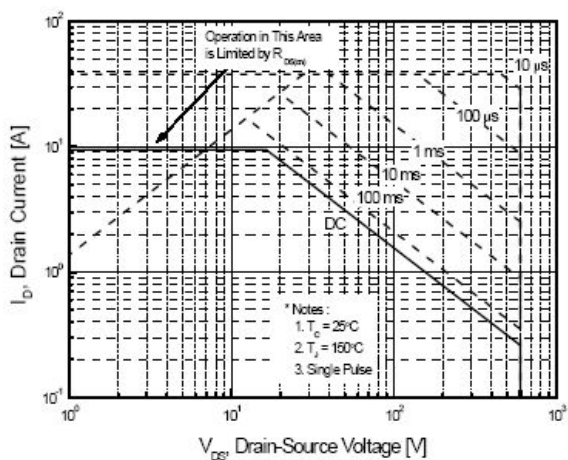
图 6-1 SIF10N60C(TO-220)
