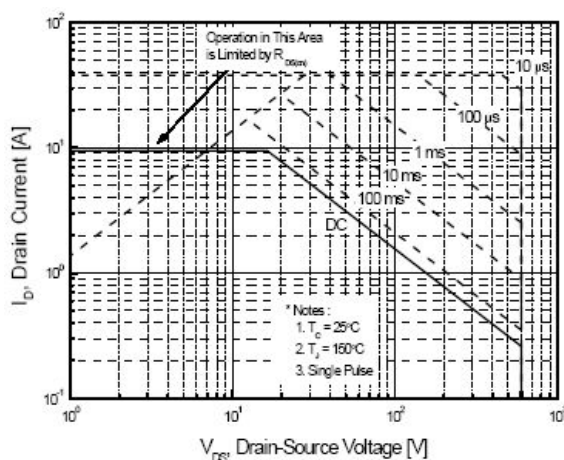
图 6-1 SIF10N60C(TO-220FP(L))
