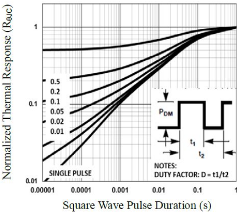
图 5 归一化阻抗
